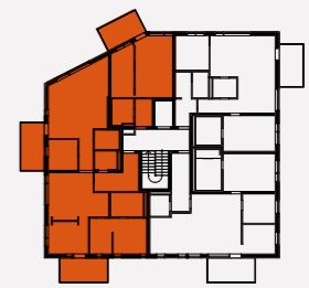
Plantegning 7. etasje
